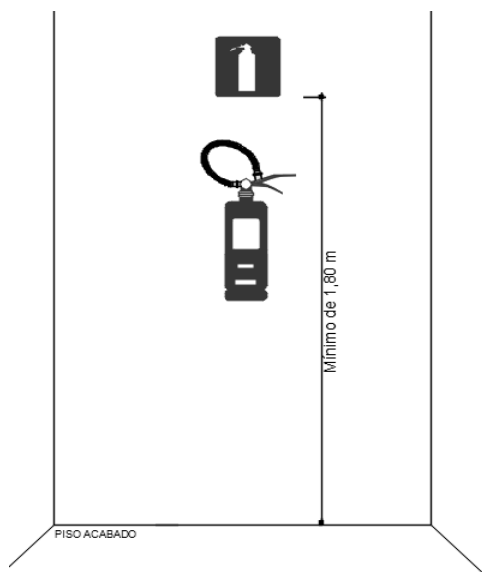
Figura 2 – Altura sinalização
