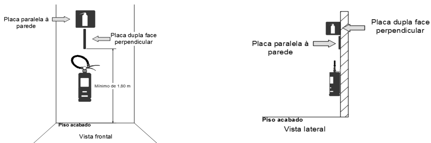
Figura 3 – Placa dupla face
