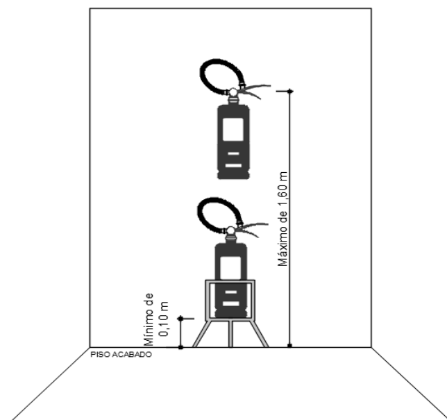
Figura 1 – Altura de instalação do extintor
